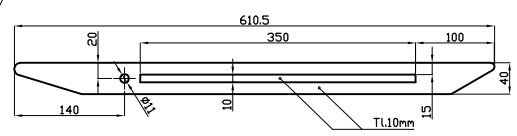
detail závory (pravá, levá)
